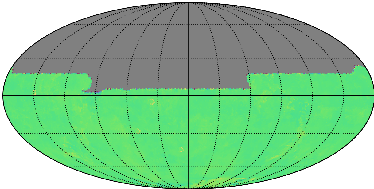
weather_cloudso1v3.4_10yrs y: Kuiper rotTelPos
