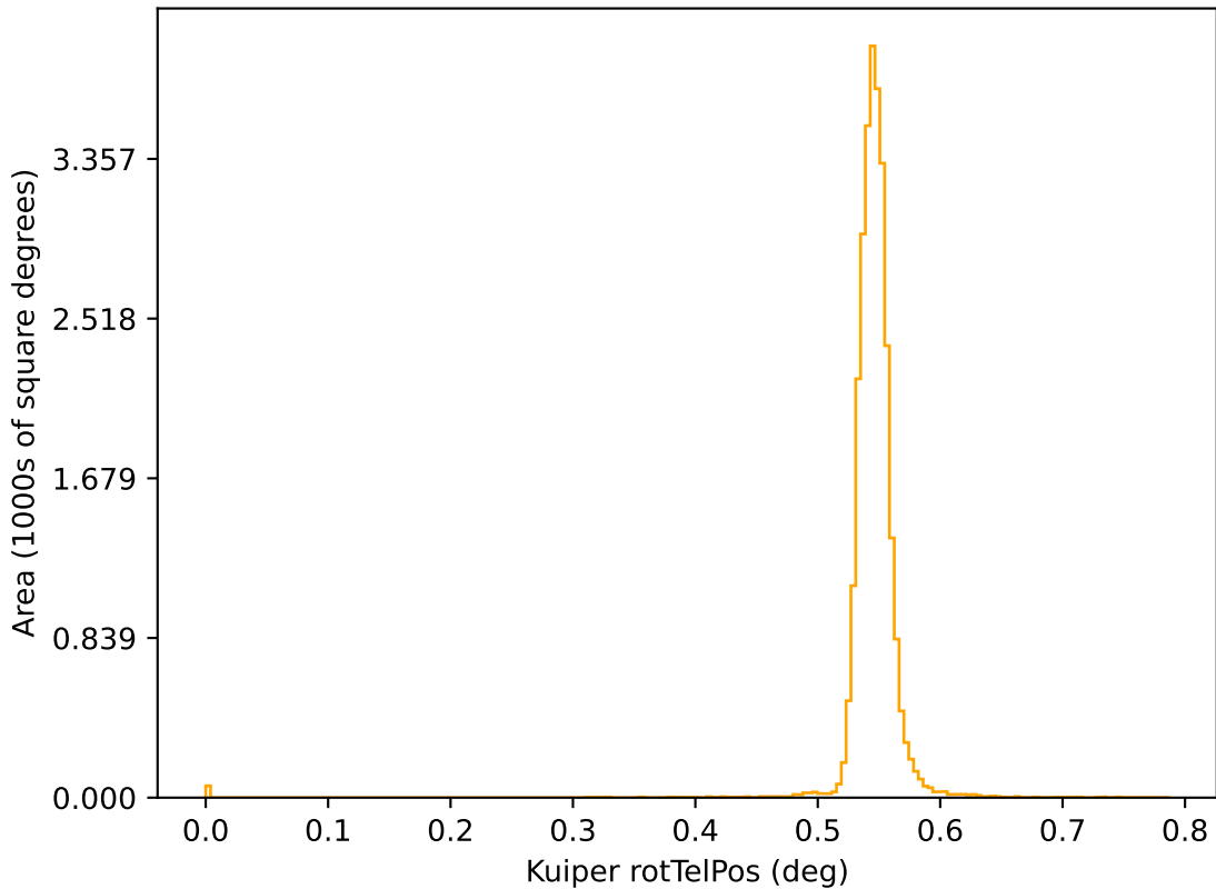
weather_cloudso1v3.4_10yrs r: Kuiper rotTelPos
