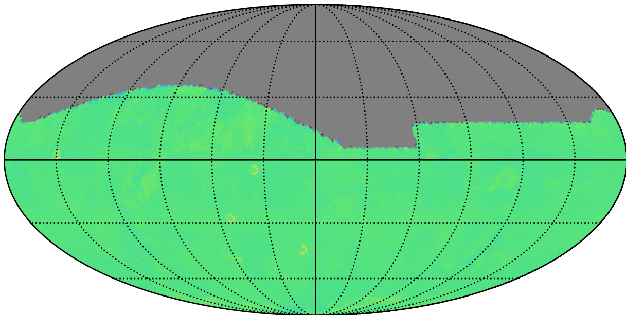
weather_cloudso1v3.4_10yrs i: Kuiper rotTelPos
