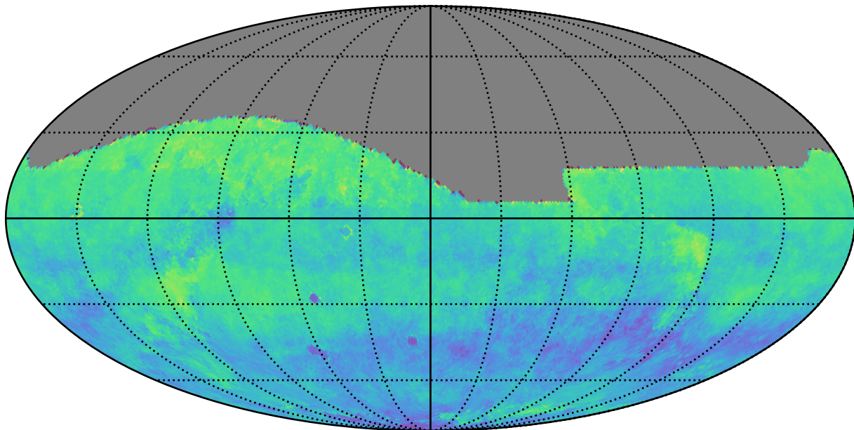
weather_cloudso1v3.4_10yrs z: Kuiper rotSkyPos
