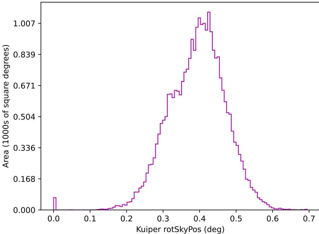
weather_cloudso1v3.4_10yrs z: Kuiper rotSkyPos
