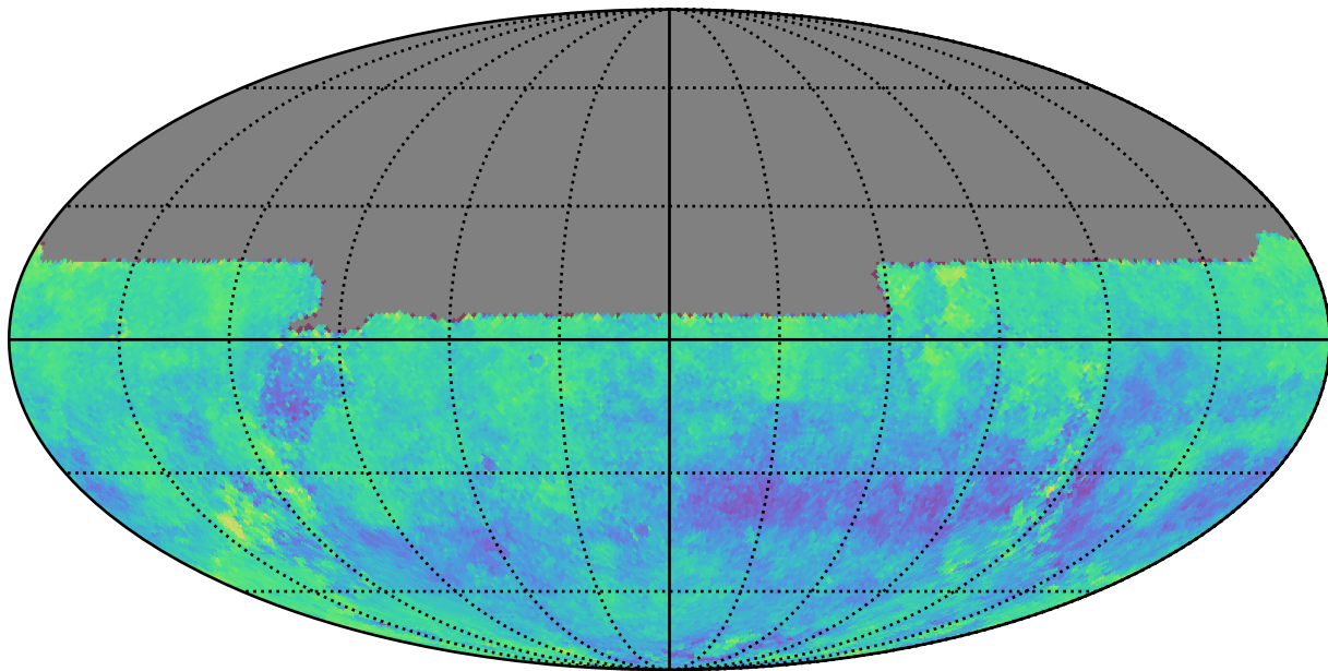
weather_cloudso1v3.4_10yrs u: Kuiper rotSkyPos
