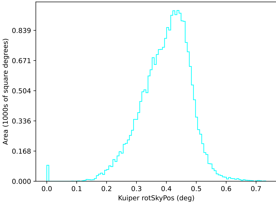
weather_cloudso1v3.4_10yrs u: Kuiper rotSkyPos
