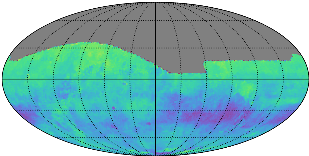
weather_cloudso1v3.4_10yrs r: Kuiper rotSkyPos
