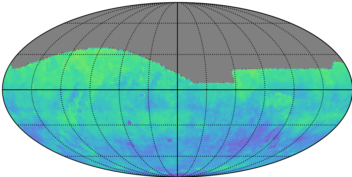
weather_cloudso1v3.4_10yrs i: Kuiper rotSkyPos
