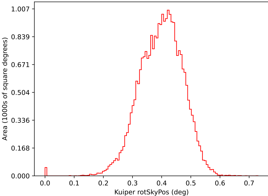
weather_cloudso1v3.4_10yrs i: Kuiper rotSkyPos
