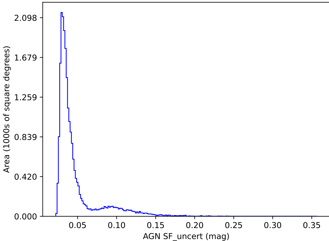
weather_cloudso1v3.4_10yrs y band: AGN SF_uncert
