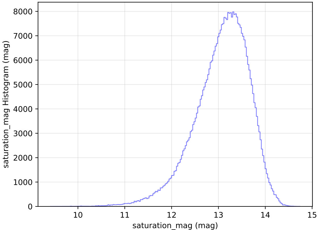
weather_cloudso1v3.4_10yrs WFD y band: saturation_mag Histogram
