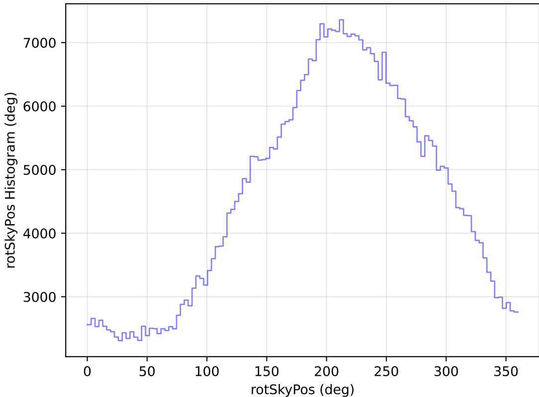
weather_cloudso1v3.4_10yrs All sky i band: rotSkyPos Histogram
