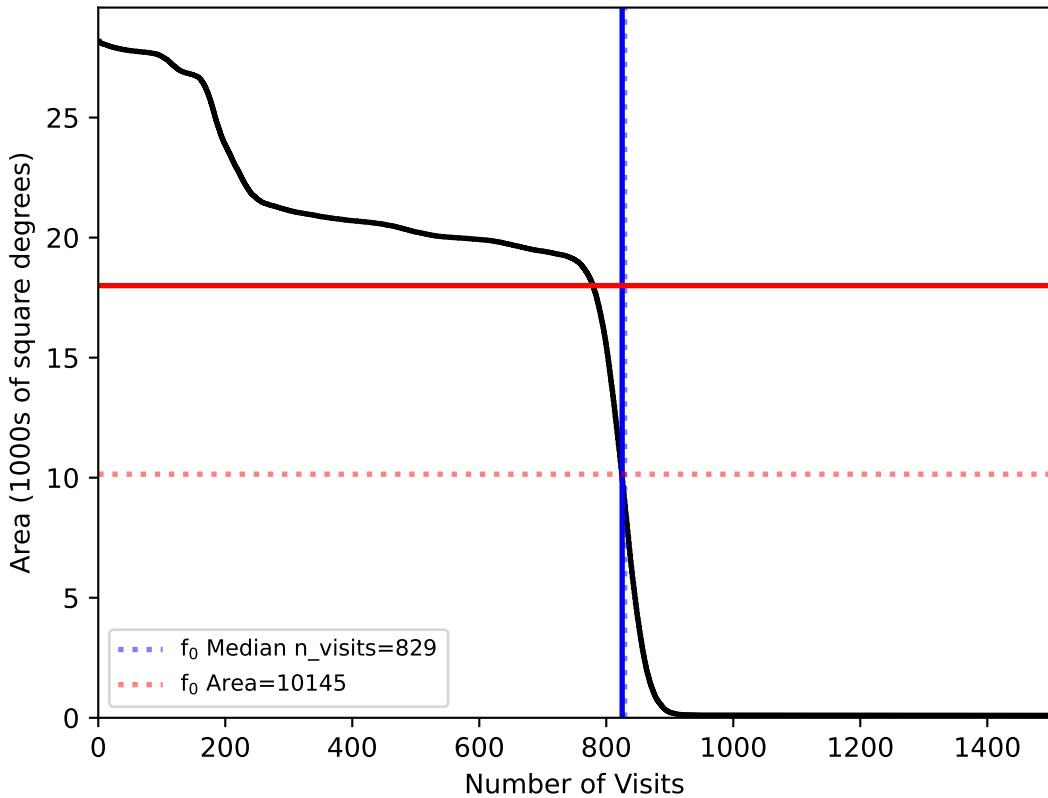
weather_cloudso1v3.4_10yrs All sky: f0
