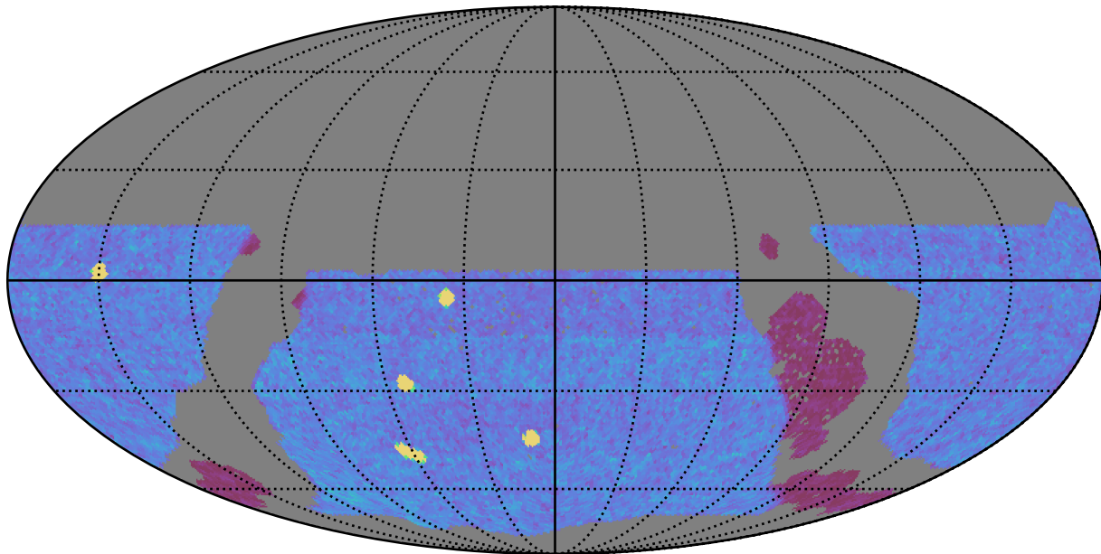
weather_cloudso1v3.4_10yrs WFD y band: NVisits
