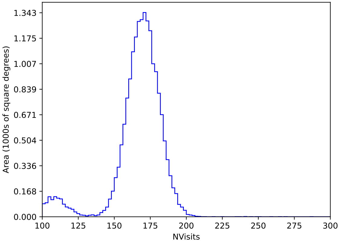
weather_cloudso1v3.4_10yrs WFD y band: NVisits
