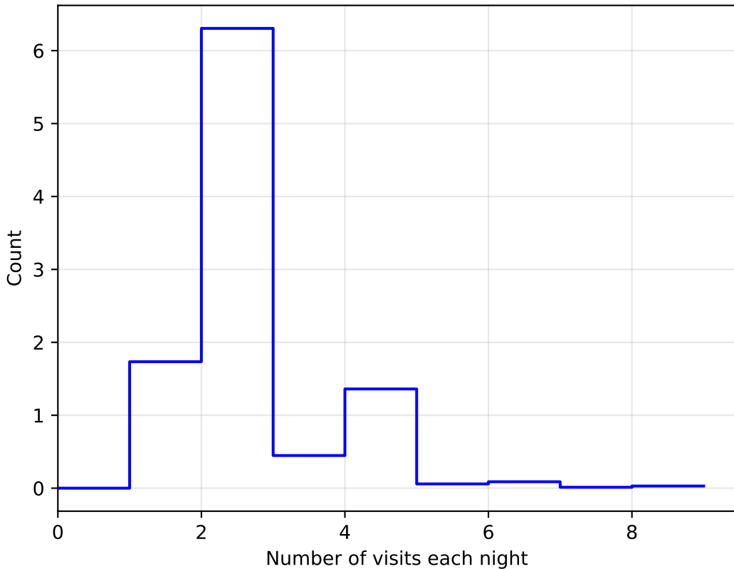
1e6 weather_cloudso1v3.4_10yrs All sky: NVisitsPerNight
