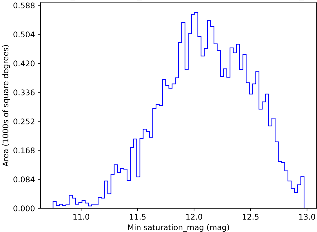
weather_cloudso1v3.4_10yrs WFD z band: Min saturation_mag
