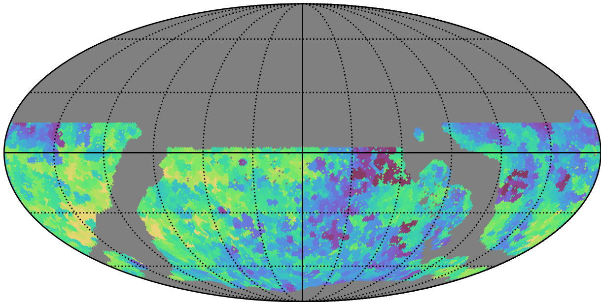
weather_cloudso1v3.4_10yrs WFD y band: Min saturation_mag
