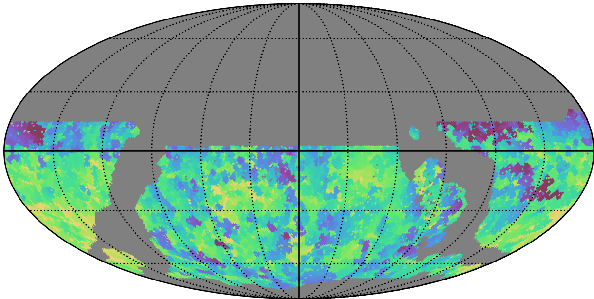
weather_cloudso1v3.4_10yrs WFD u band: Min saturation_mag
