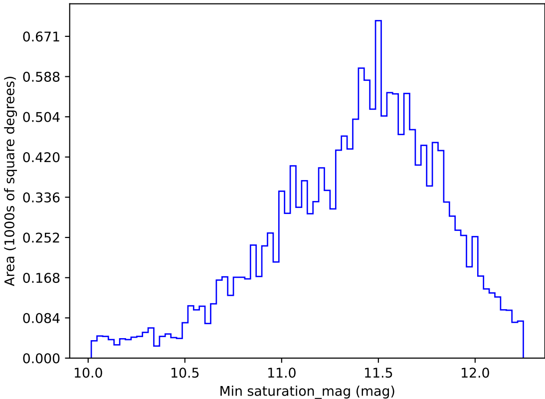
weather_cloudso1v3.4_10yrs WFD u band: Min saturation_mag
