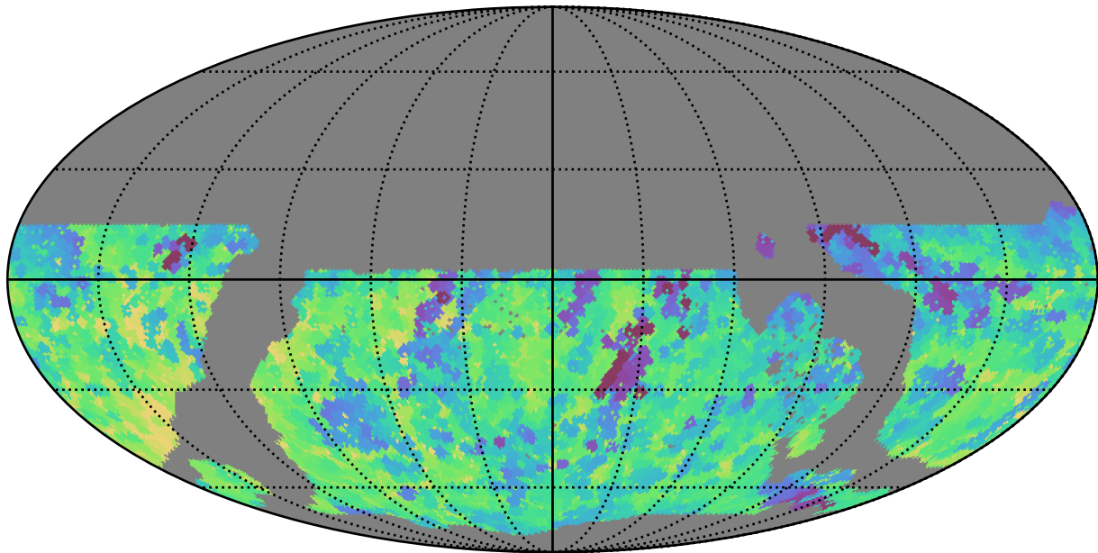
weather_cloudso1v3.4_10yrs WFD r band: Min saturation_mag
