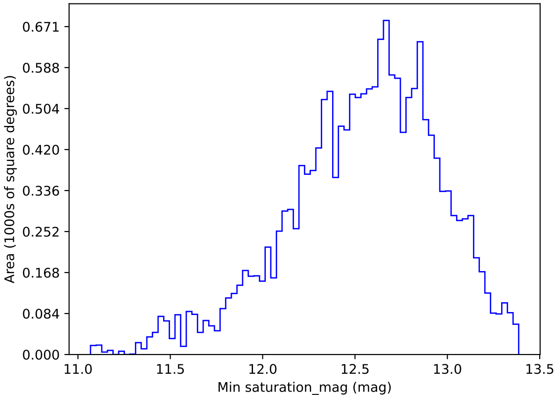
weather_cloudso1v3.4_10yrs WFD r band: Min saturation_mag
