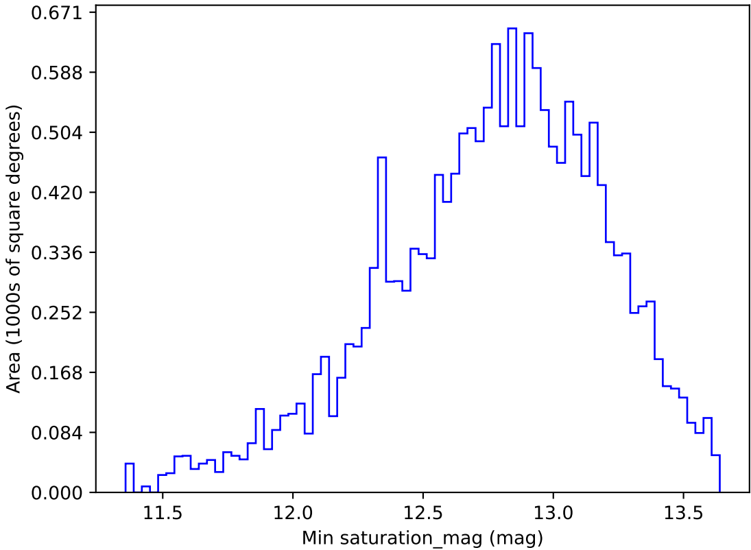
weather_cloudso1v3.4_10yrs WFD g band: Min saturation_mag
