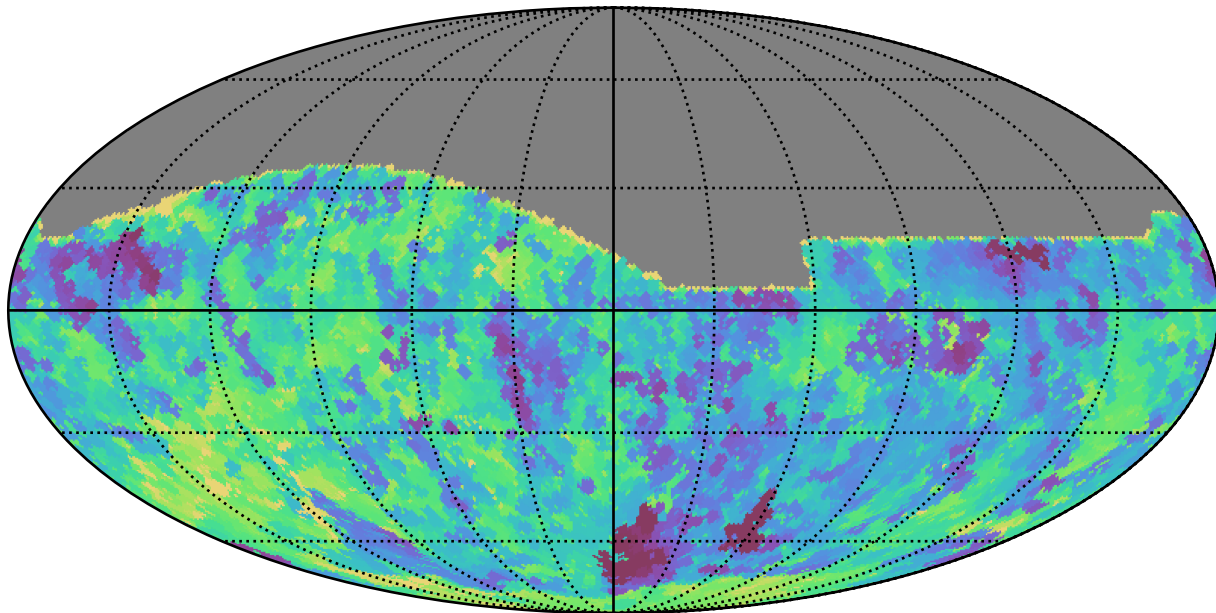
weather_cloudso1v3.4_10yrs All sky z band: Min saturation_mag
