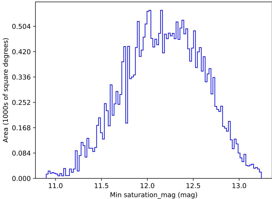
weather_cloudso1v3.4_10yrs All sky z band: Min saturation_mag
