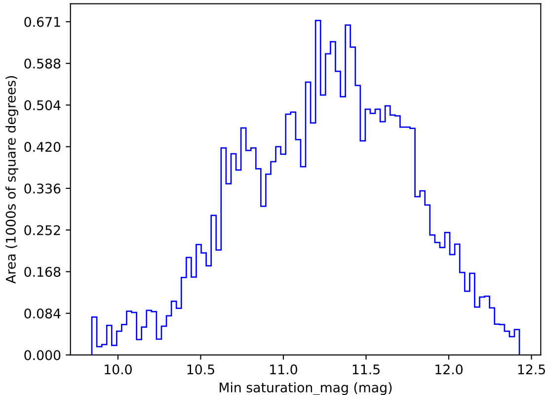
weather_cloudso1v3.4_10yrs All sky y band: Min saturation_mag
