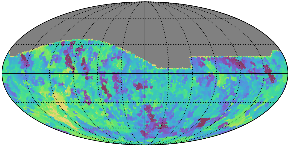
weather_cloudso1v3.4_10yrs All sky i band: Min saturation_mag
