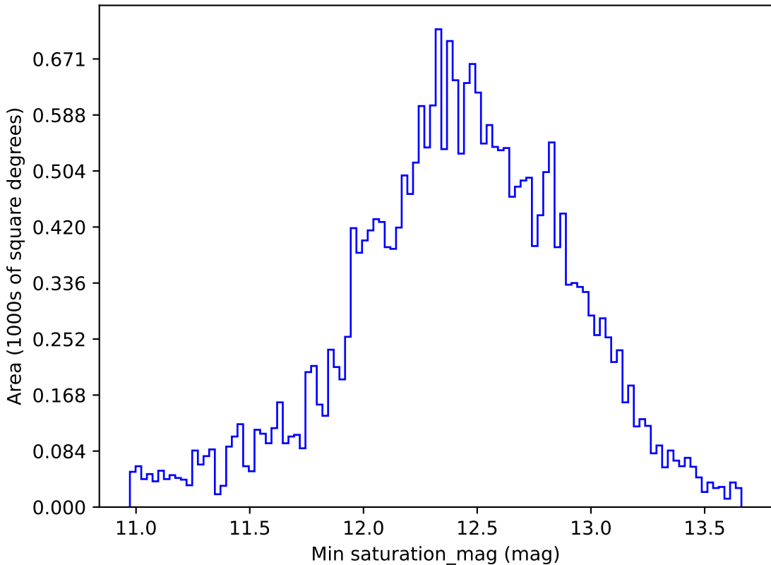
weather_cloudso1v3.4_10yrs All sky i band: Min saturation_mag
