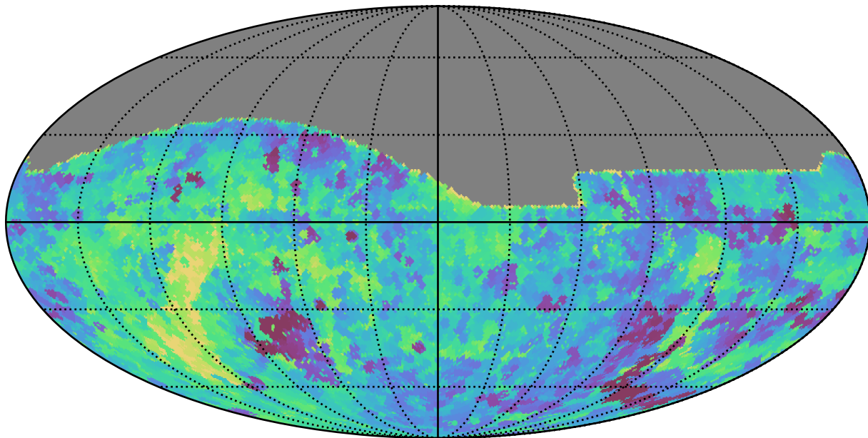
weather_cloudso1v3.4_10yrs All sky g band: Min saturation_mag
