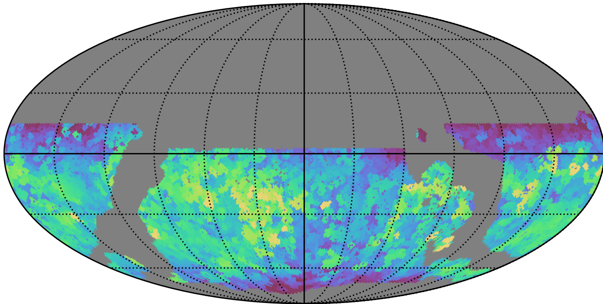
weather_cloudso1v3.4_10yrs WFD i band: Max saturation_mag
