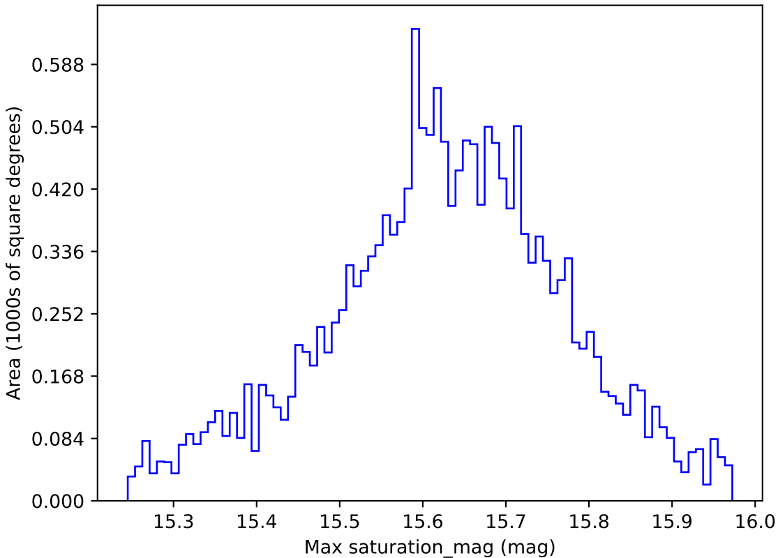
weather_cloudso1v3.4_10yrs WFD i band: Max saturation_mag
