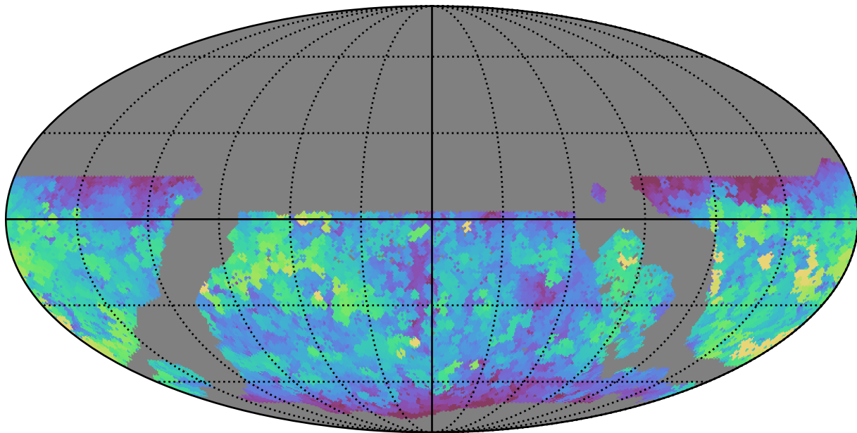
weather_cloudso1v3.4_10yrs WFD g band: Max saturation_mag
