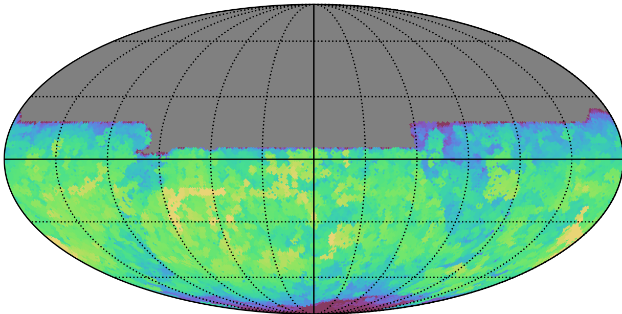
weather_cloudso1v3.4_10yrs All sky y band: Max saturation_mag
