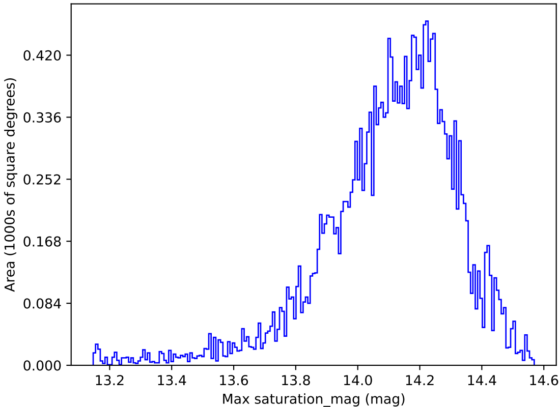
weather_cloudso1v3.4_10yrs All sky y band: Max saturation_mag
