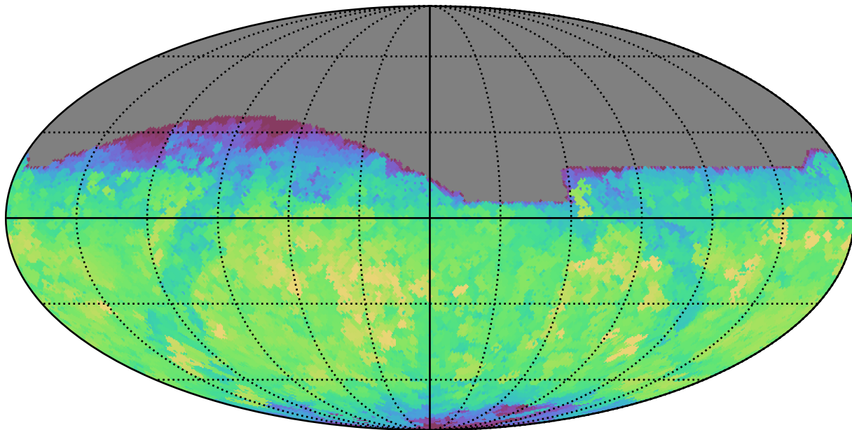
weather_cloudso1v3.4_10yrs All sky i band: Max saturation_mag
