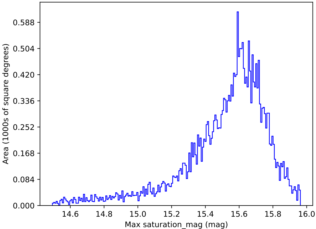
weather_cloudso1v3.4_10yrs All sky i band: Max saturation_mag
