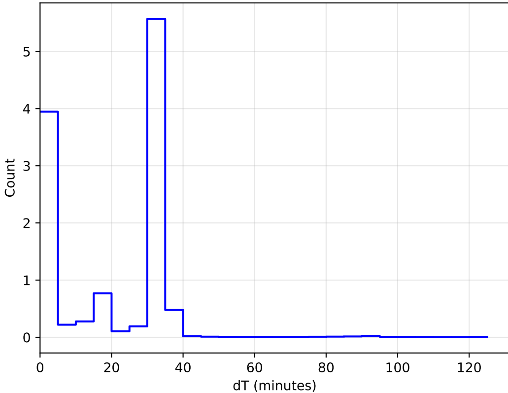
weather_cloudso1v3.4_10yrs WFD: DeltaT Histogram
