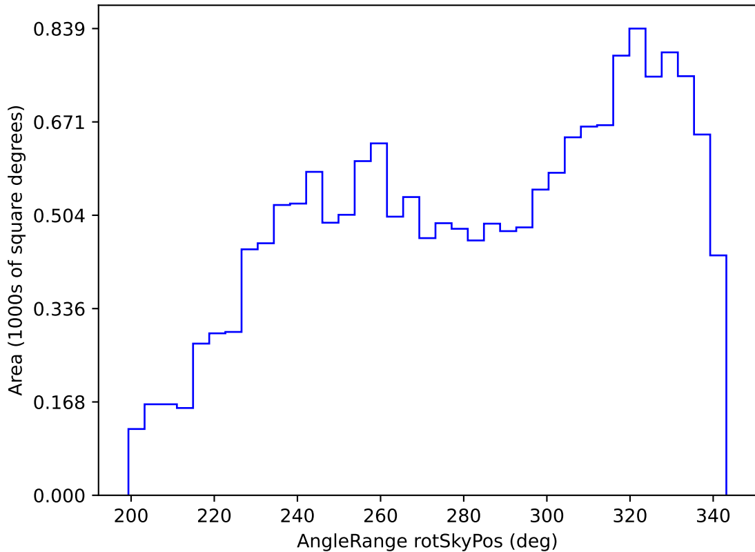
weather_cloudso1v3.4_10yrs WFD z band: AngleRange rotSkyPos
