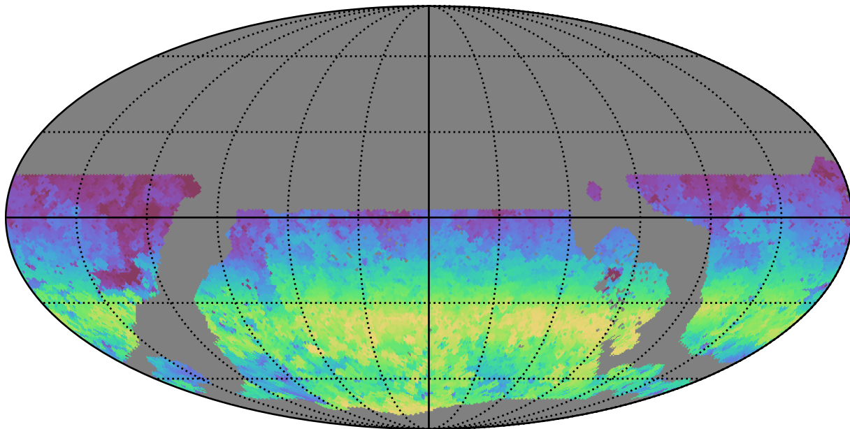
weather_cloudso1v3.4_10yrs WFD y band: AngleRange rotSkyPos
