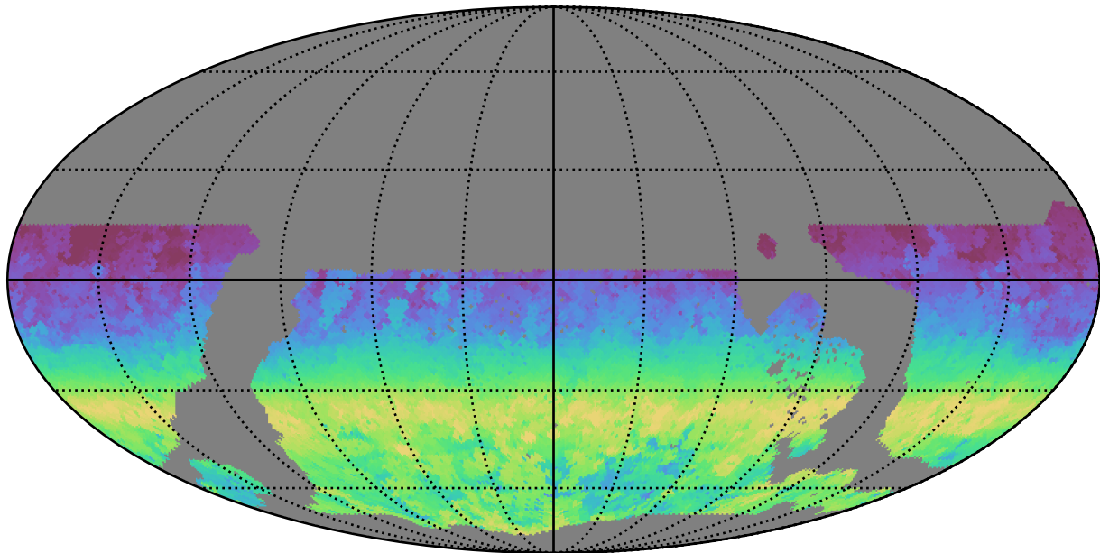
weather_cloudso1v3.4_10yrs WFD r band: AngleRange rotSkyPos
