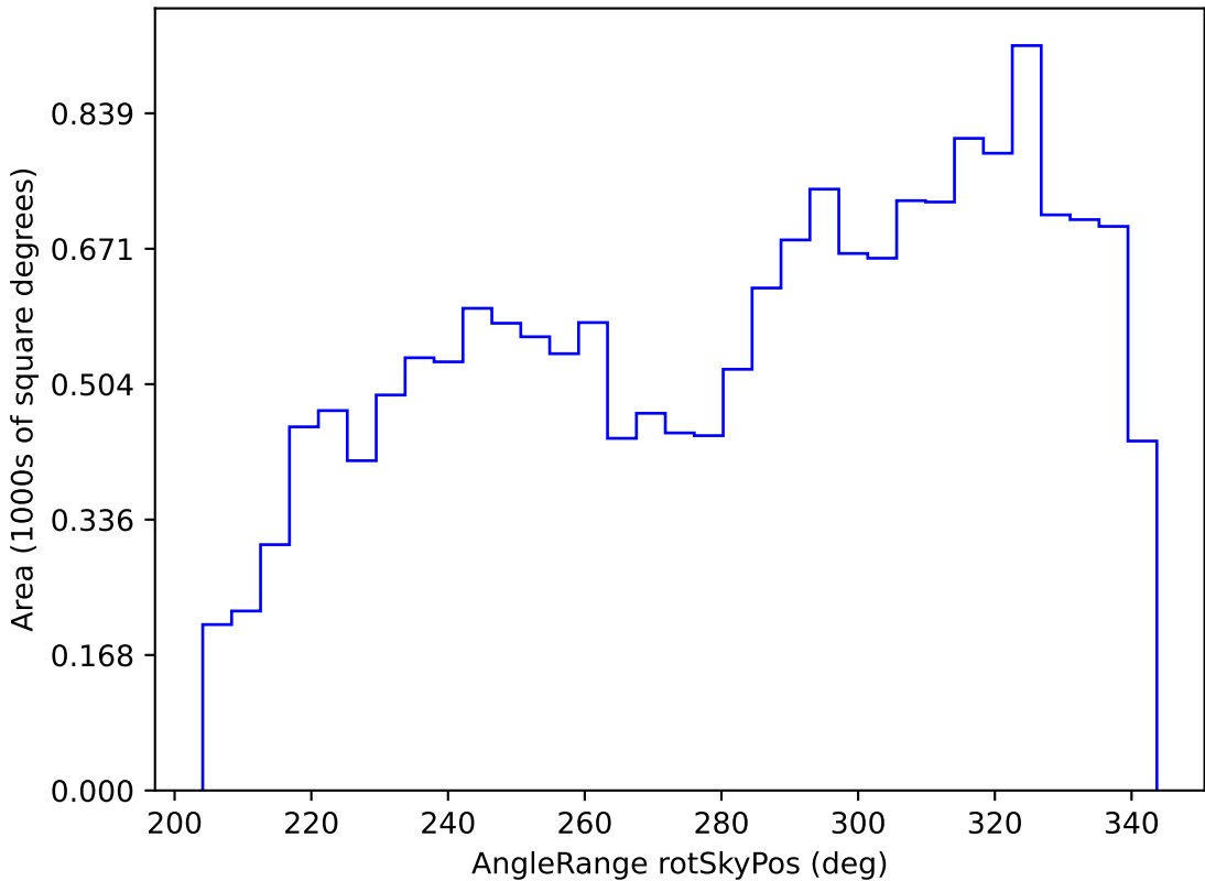
weather_cloudso1v3.4_10yrs WFD r band: AngleRange rotSkyPos
