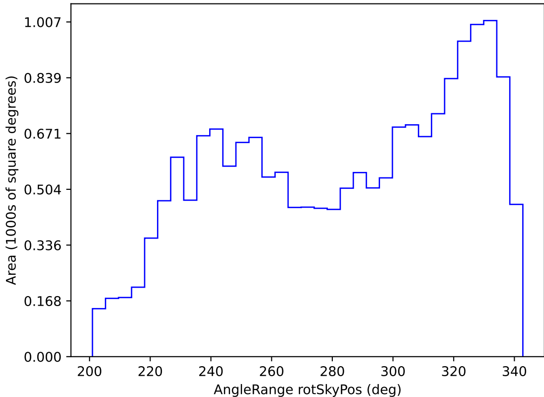
weather_cloudso1v3.4_10yrs WFD i band: AngleRange rotSkyPos
