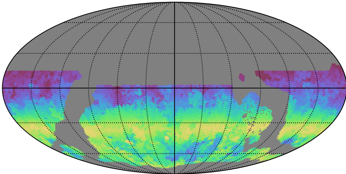
weather_cloudso1v3.4_10yrs WFD g band: AngleRange rotSkyPos
