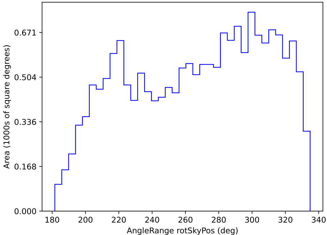
weather_cloudso1v3.4_10yrs WFD g band: AngleRange rotSkyPos
