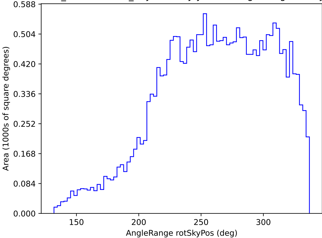
weather_cloudso1v3.4_10yrs All sky y band: AngleRange rotSkyPos
