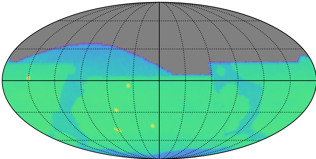
weather_cloudso1v3.4_10yrs i: CoaddM5
