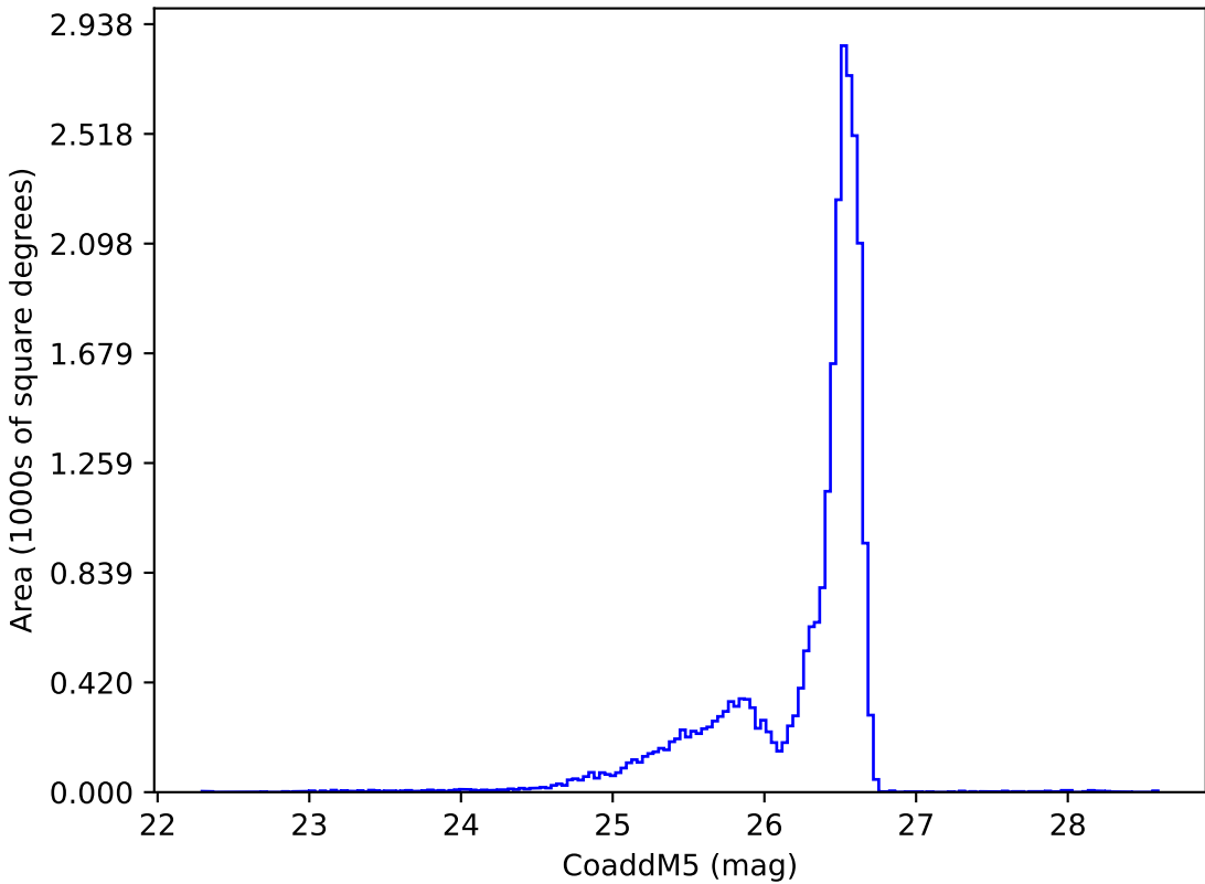
weather_cloudso1v3.4_10yrs i: CoaddM5
