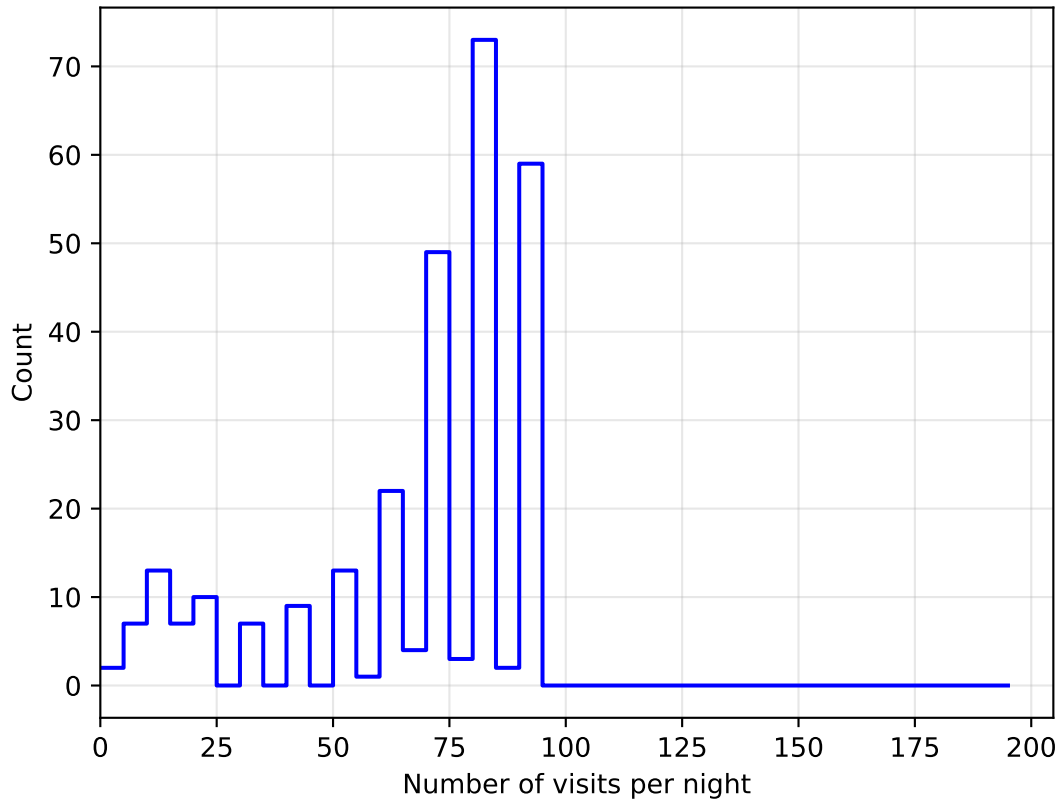
weather_cloudso1v3.4_10yrs all bands: DD:ELAISS1 NVisitsPerNight
