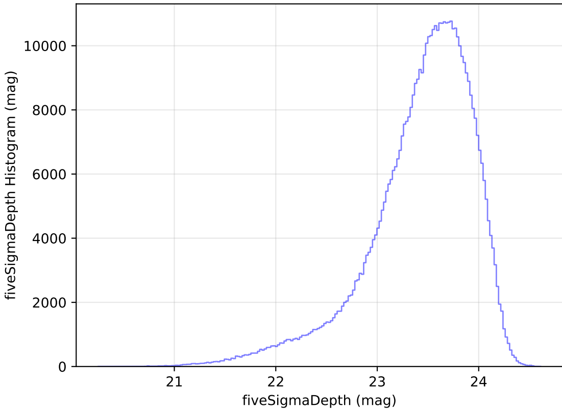
weather_cloudso18v3.4_10yrs i: fiveSigmaDepth Histogram
